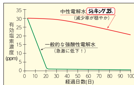
【図2】有効塩素濃度変化
