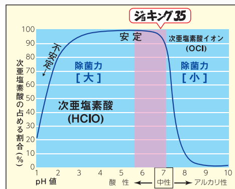
【図1】pH値と次亜塩素酸含有率(%)
